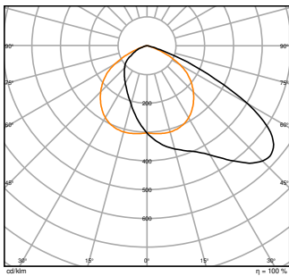
FL PFM DA 200W 3000K ASYM 55X110 BK
