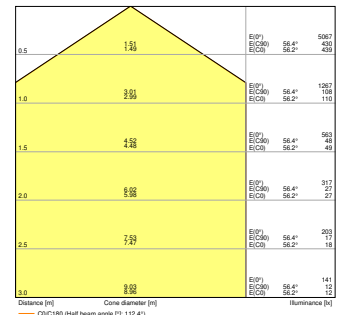
PL CMFT 625 P 28W 840 DALIVR
